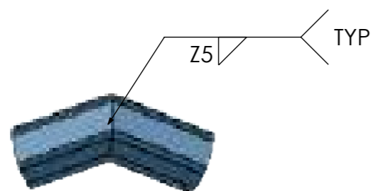
DETAIL AY SCALE 1 : 7
