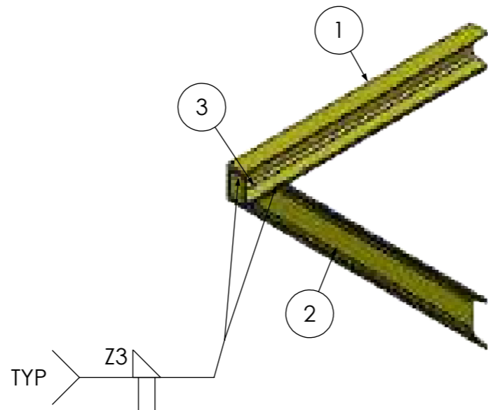
DETAIL AB SCALE 1 : 10
