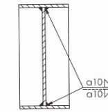
SECTION AN-AN SCALE 1 : 10
