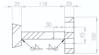
A-A (1 : 3)
