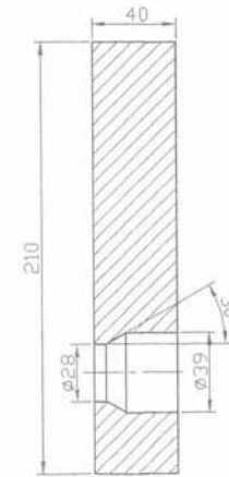
SECTION A-A SCALE 1:2
